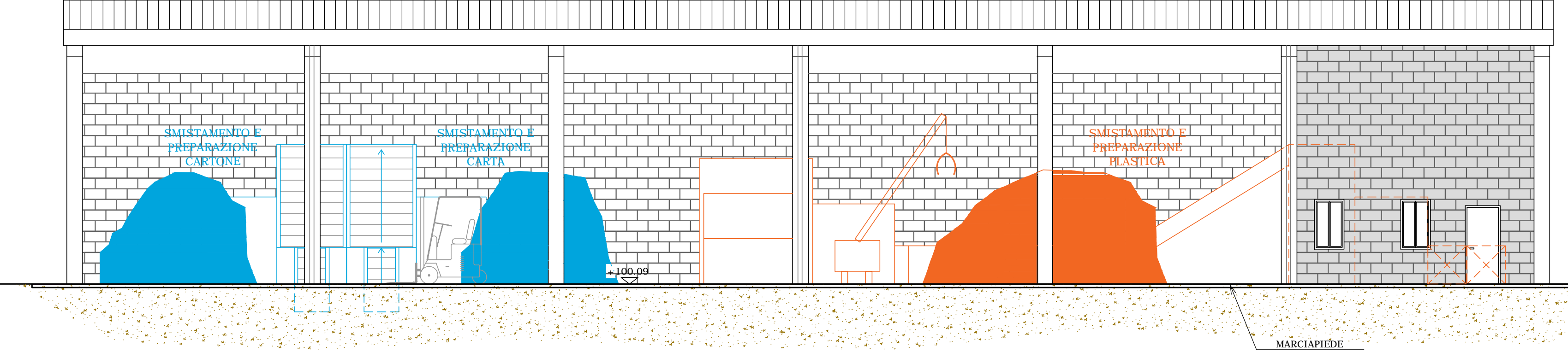
PROSPETTO SUD-OVEST Scala 1: 100
